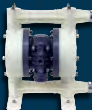
NDP-25 Полипропилен- внутренняя коническая резьба Габариты: 366 мм x 429 мм Вес нетто: 10,9 кг Вес брутто: 12,6 кг
